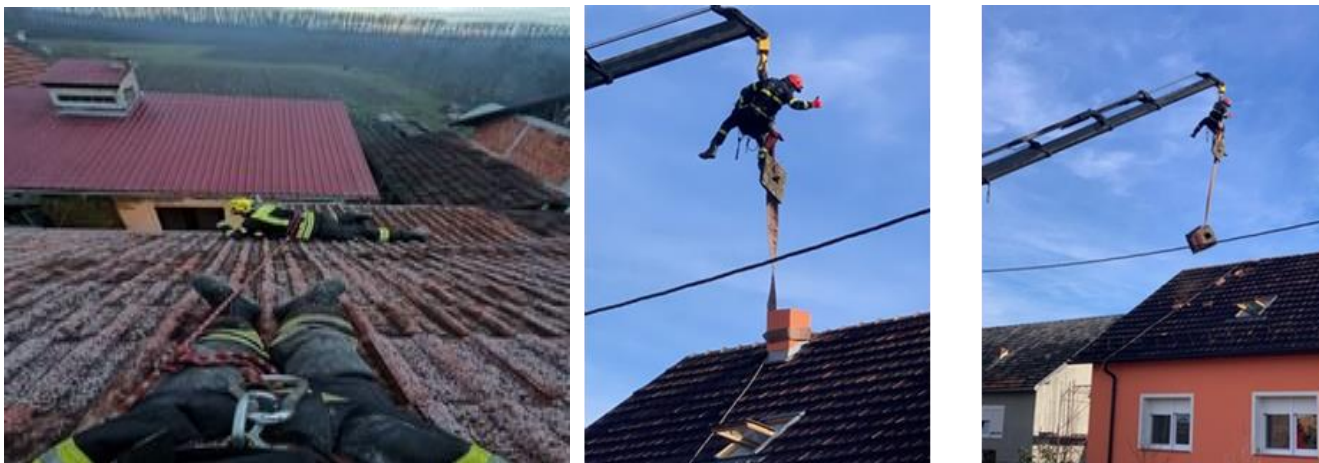
Detalj skidanja dimnjaka i rubnih dijelova krovišta
